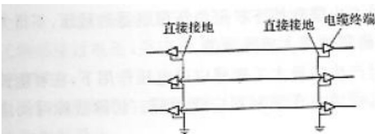
图 4.1.11-2 线路两端直接接地
